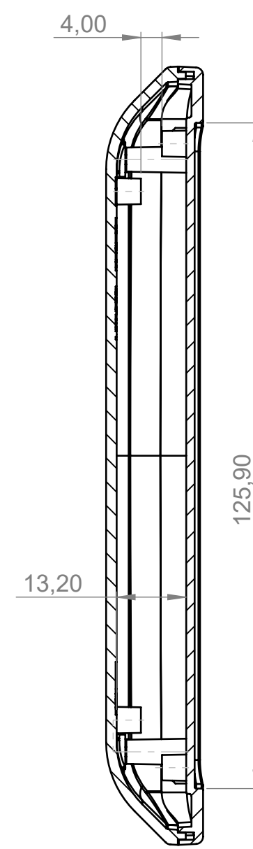
Schnitt A-A
