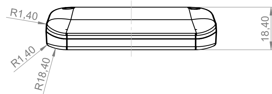
Schnitt B-B
