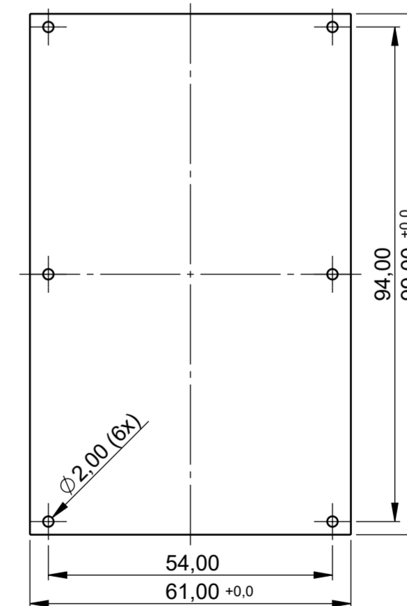
Platine Oberteil PCB top
