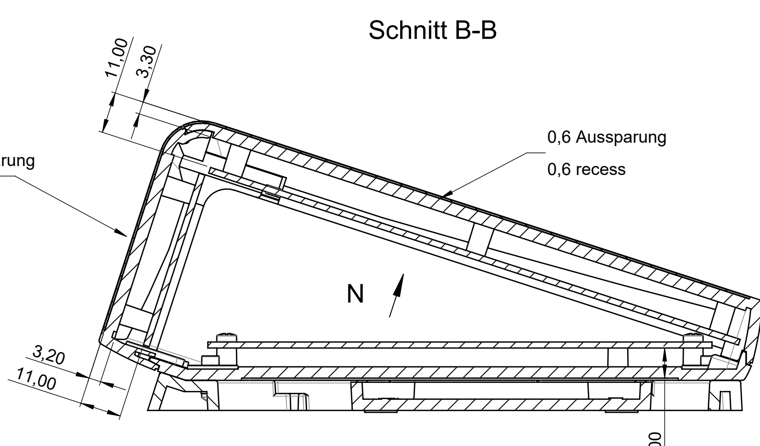
Hauptteil mit Wandmontage Main section with wall mounting
