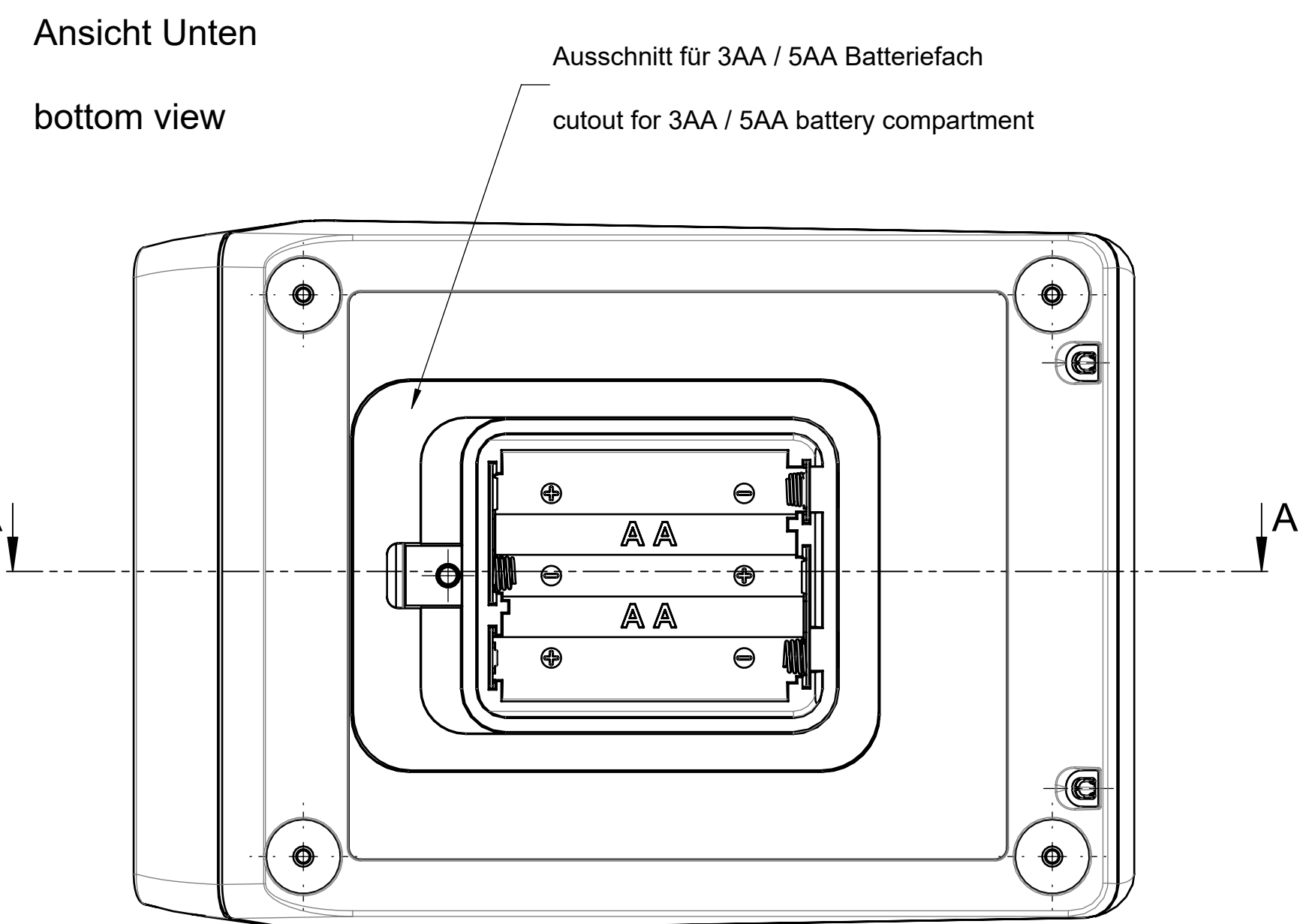
Hauptteil mit Batteriefach Main section with battery compartment
