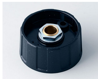
A2531060 Круглая ручка 31, без риски АБС (UL 94 HB) черный RAL 9005 31x15mm 6mm
