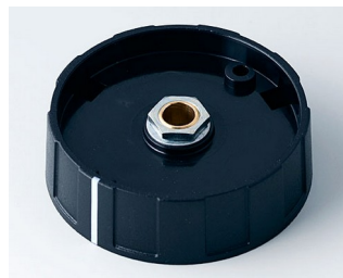
A2650060 Круглая ручка 50, с риской АБС (UL 94 HB) черный RAL 9005 50x15mm 6mm
