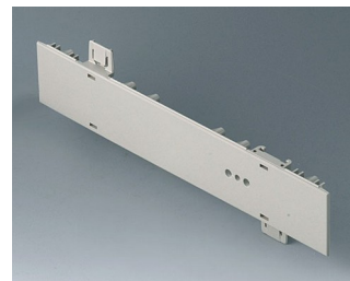
A0111280 Боковая панель для 1 U с отверстиями для крепления ручки АБС (UL 94 HB) тепло-серый RAL 7032 250x44,45mm
