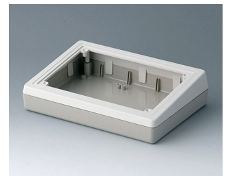
A9086265 DESK CASE 190 F ABC (UL 94 HB) тепло-серый RAL 7032 190x138x47mm
