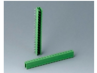
B6604222 Вилочная часть соединителя, шаг 5,08 мм ПА 68 (UL 94 V-0)
