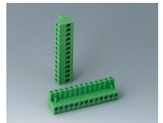
B6605223 Розеточная часть соединителя, шаг 5,08 мм ПА 6 (UL 94 V-0)
