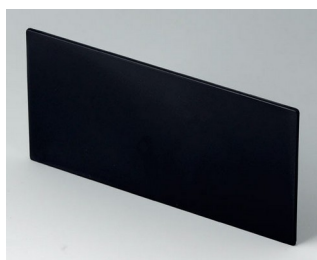
B6143221 Лицевая панель PPO (UL 94 V-0) черный RAL 9005 139,3x67,5x2mm
