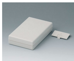
A9408335 SHELL-TYPE CASE G 155, исп. IV АБС (UL 94 HB) белый RAL 9002 95x158x33mm
