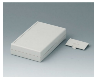
A9408355 SHELL-TYPE CASE G 155, исп. IV АБС (UL 94 HB) белый RAL 9002 95x158x33,5mm
