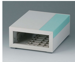
B2213015 MEDITEC E 160, без ручки ABC (UL 94 HB) белый RAL 9002 160x200x74mm IP 40
