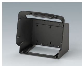
C3602708 COMMUNITEC S, basic housing ACA+ПК (UL 94 V-0) тёмно-серый RAL 7016 280x169x242mm IP 40
