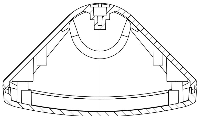
Schnitt B-B
