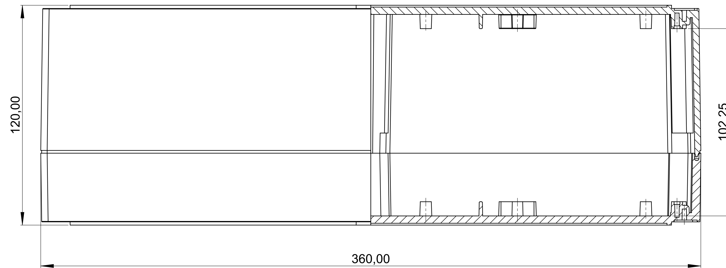
Schnitt B-B
