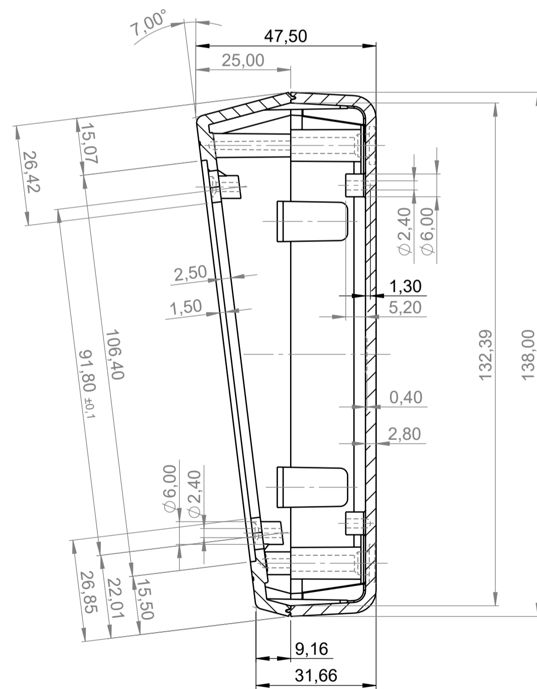
Schnitt A-A
