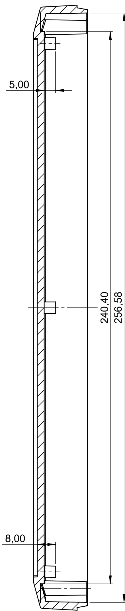
Schnitt B-B
