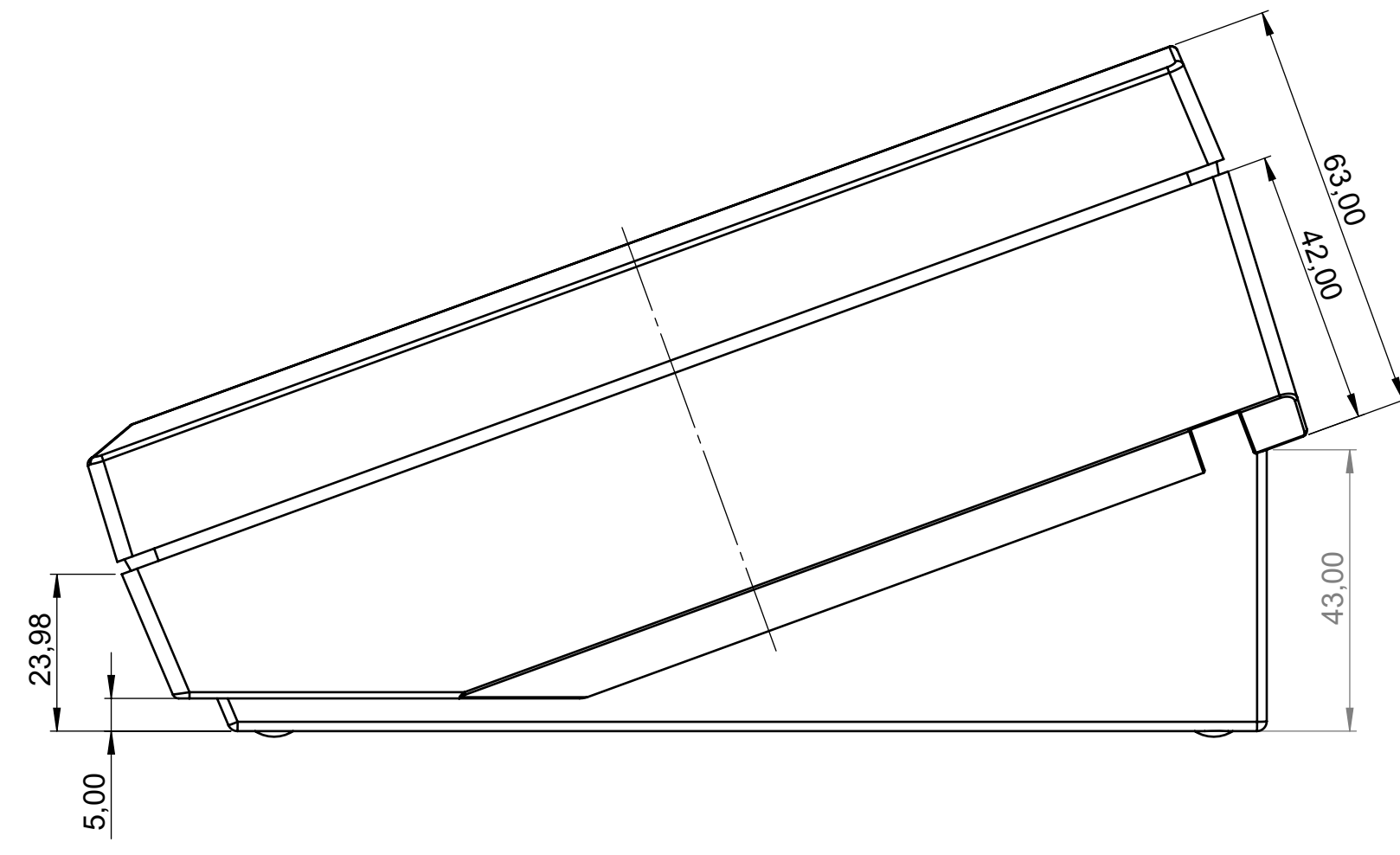
Schnitt B-B
