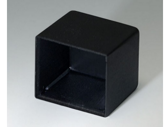
A8017158 BOITIER VIDE POUR MODULES, Vers. II PA 66 (UL 94 HB) noir RAL 9005 17,4x15x15,3mm
