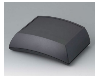
B7025209 ERGO-CASE L, surélévée ABS (UL 94 HB) noir RAL 9005 150x200x69mm IP 54 opt.
