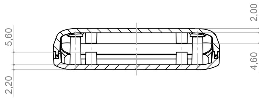
Schnitt B-B
