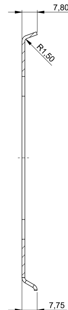
Schnitt B-B
