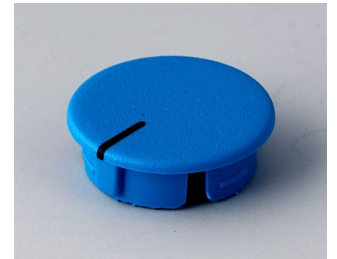
A4116106 Deckel 16, mit Strich ABS (UL 94 HB) lichtblau RAL 5012
