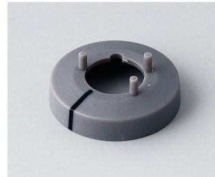
A7510018 Mutterabdeckung 10, mit Strich ABS (UL 94 HB) staubgrau RAL 7037
