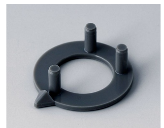
A4220008 Pfeilscheibe 20 ABS (UL 94 HB) staubgrau RAL 7037
