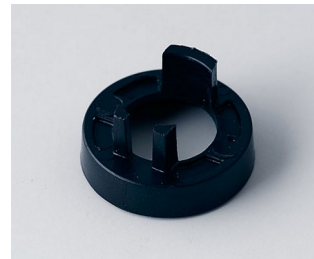
A5116000 Mutterabdeckung 16, ohne Strich ABS (UL 94 HB) schwarz RAL 9005
