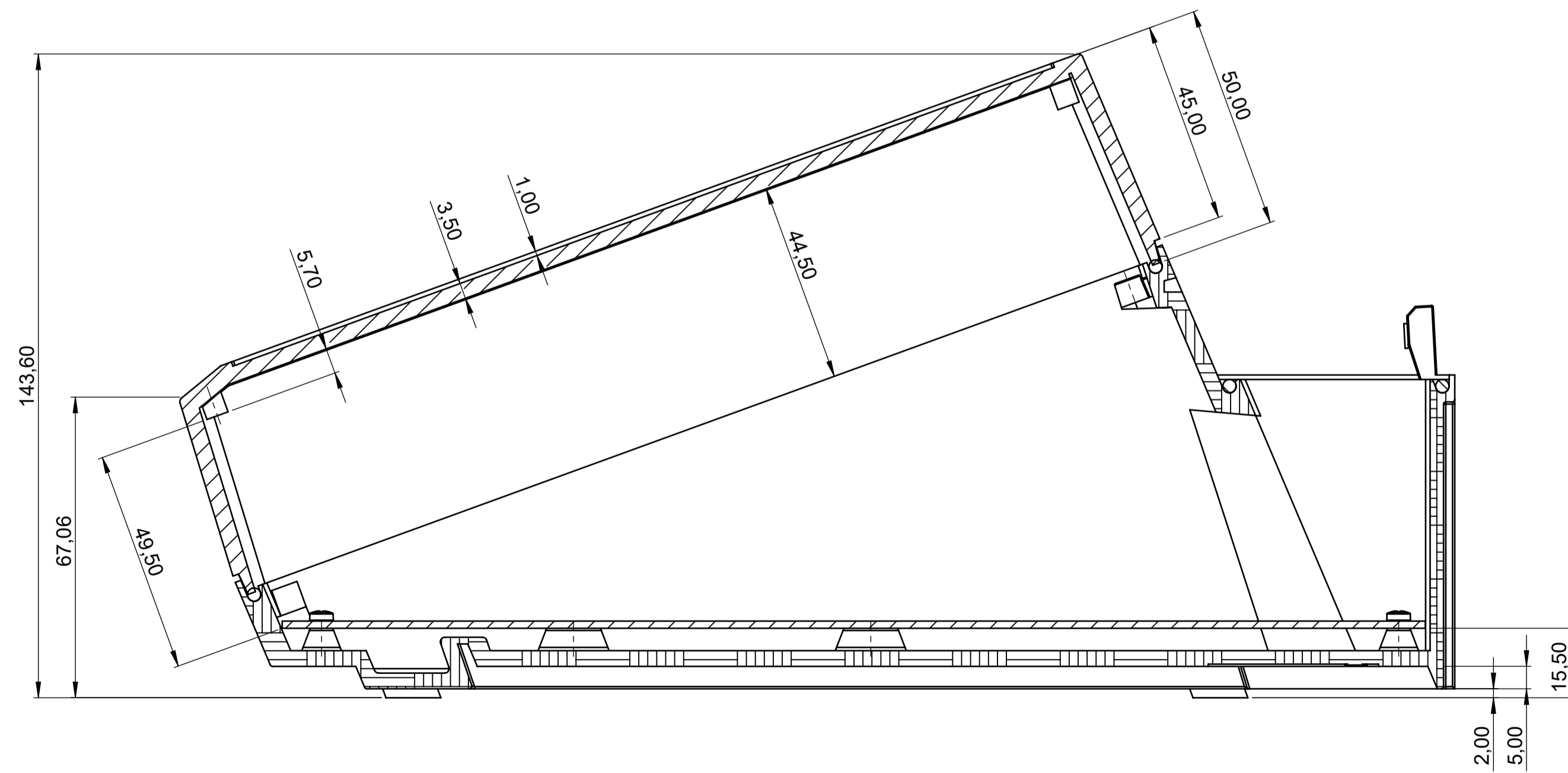
Schnitt B-B
