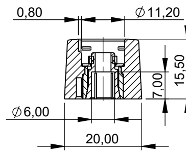
Schnitt B-B
